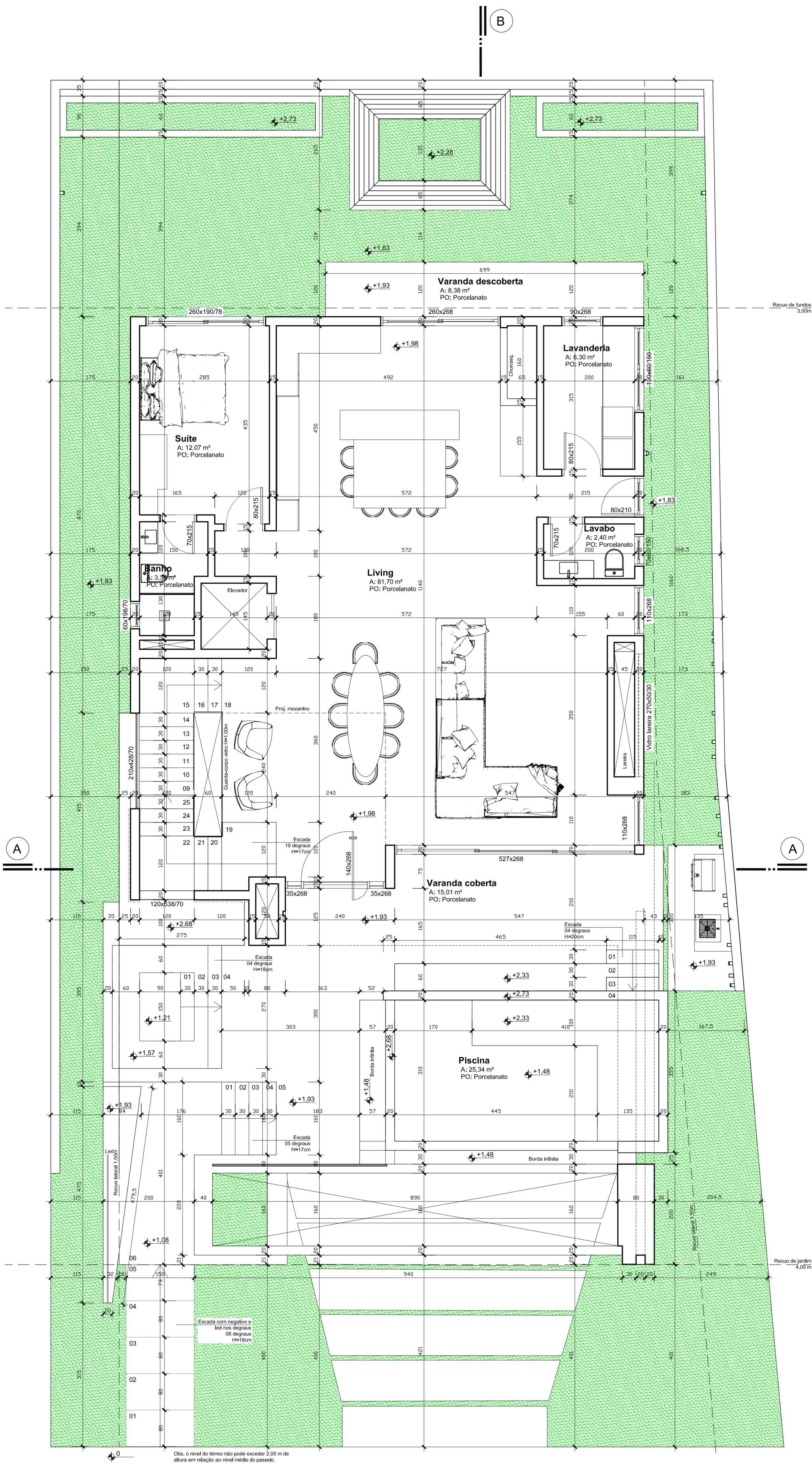
Planta Baixa Térreo Área: 150,15 m 2 Piscina: 25,34 m 2 Esc. 1/50
